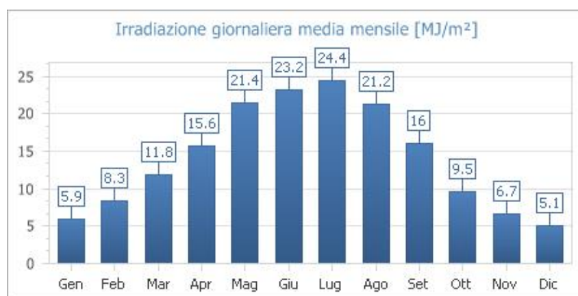
Fig. 1: Irradiazione giornaliera media mensile sul piano orizzontale [MJ/m 2 ]- Fonte dati: UNI 10349:2016 - Stazione di rilevazione: San Giuliano Terme - Metato
